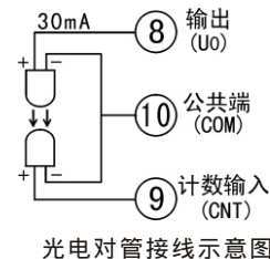
光电对管接线示意图
